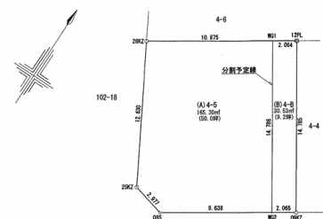
分割計画図 八戸市長根一丁目
